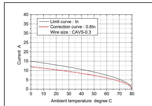
Figure-2 Derating curve 軽減曲線
