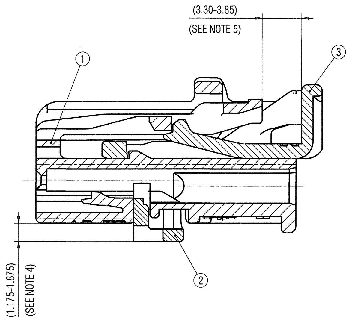
SECTION A-A
