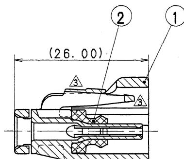
SEC. A-A
