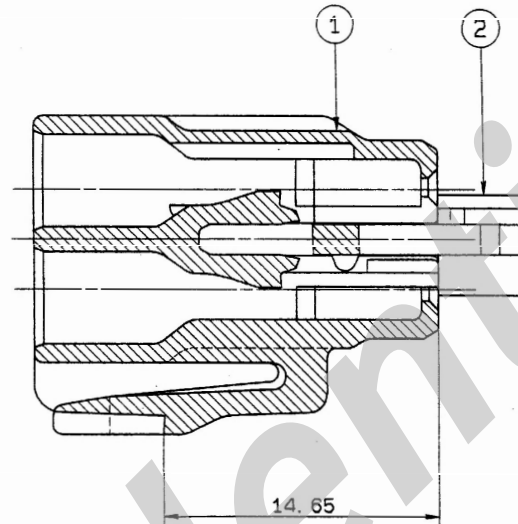
SEC. A-A
