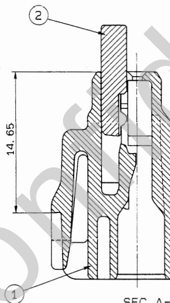
SEC. A-A
