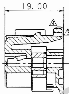
SEC. A-A
