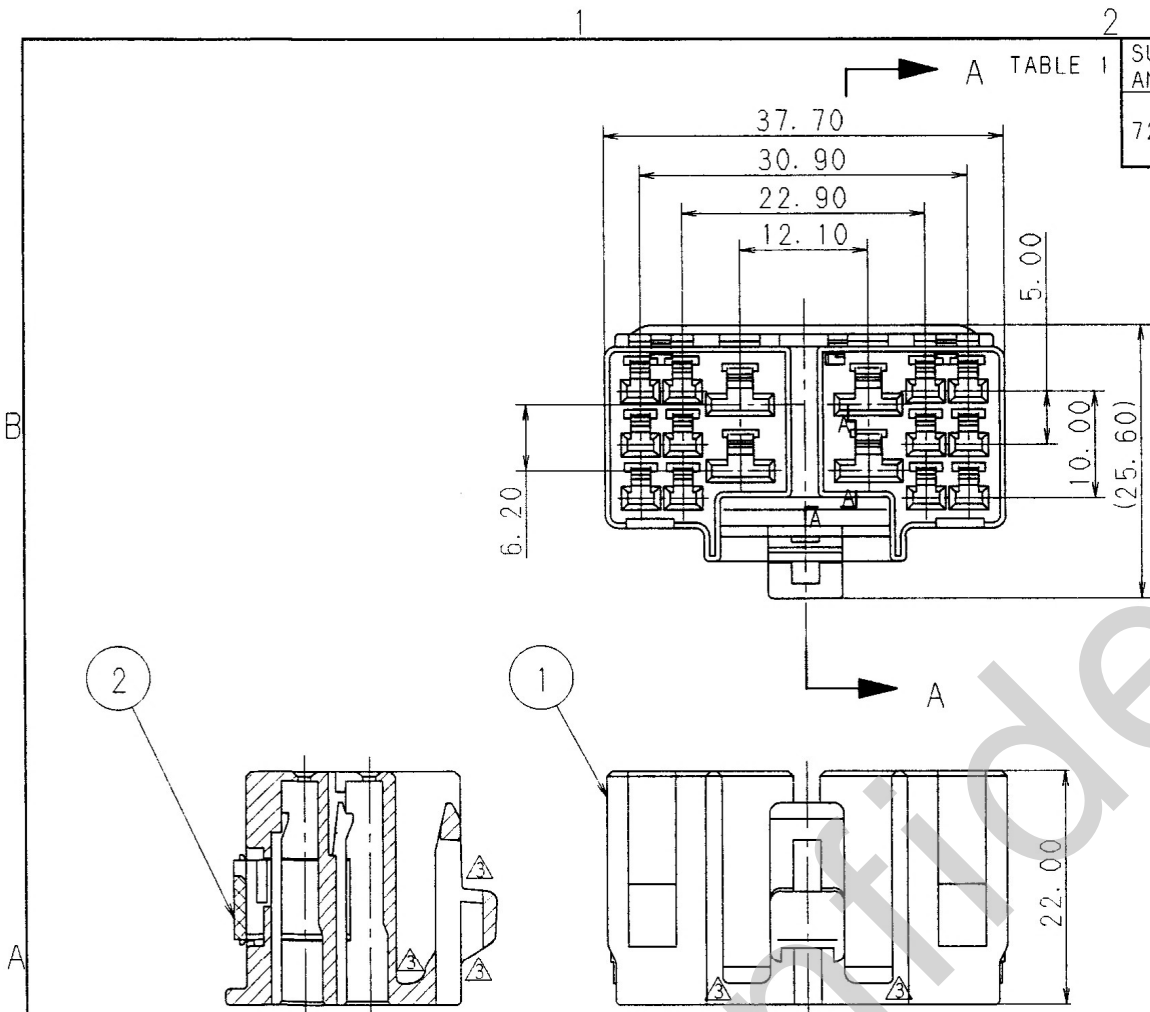
SEC. A-A
