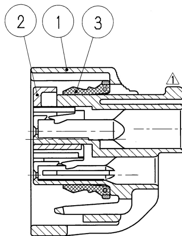
SEC. A-A
