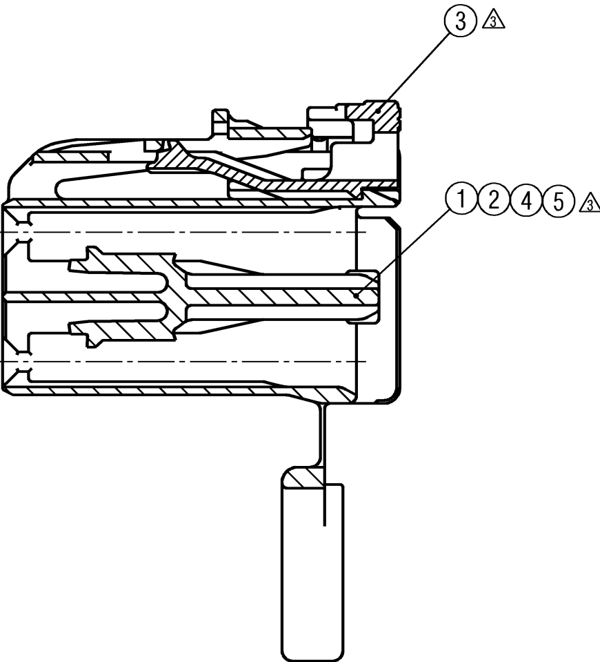
SECTION A-A (SCALE 2:1)
