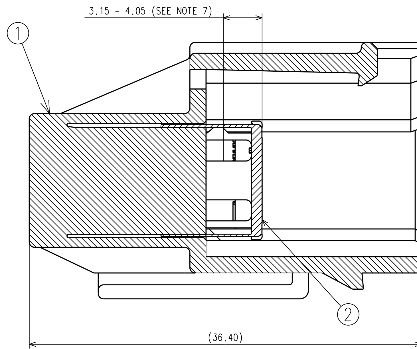
SECTION A-A
