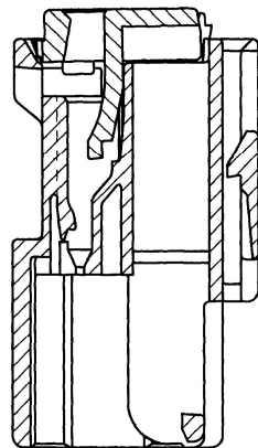
SEC. A-A
