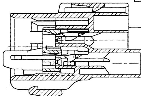
SEC. A-A
