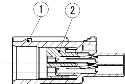
SEC. A-A
