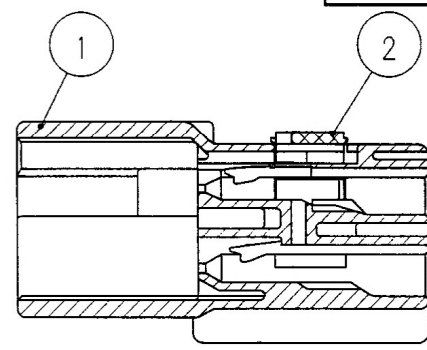
SEC. A-A
