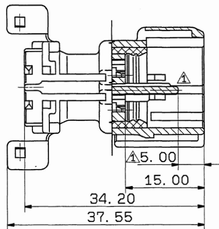
△SEC. A-A
