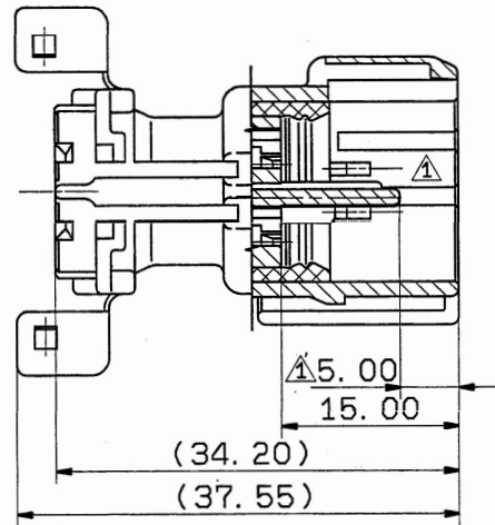
SEC. A-A
