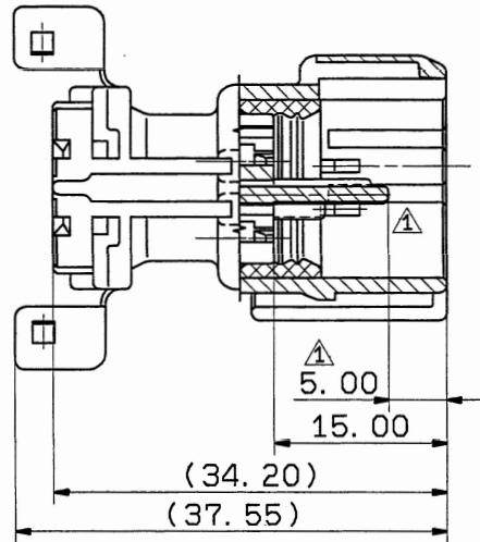
△ SEC. A-A
