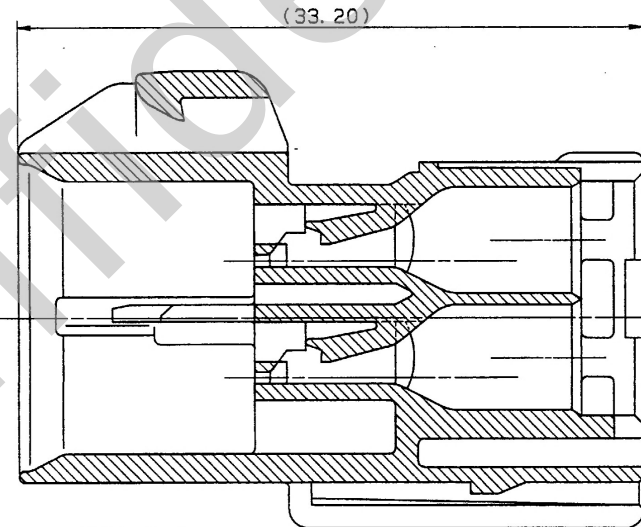
SEC. A-A
