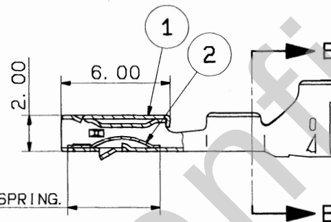
SEC. A-A
